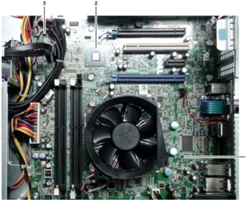
Kuva 2. Emolevy ilman lämpöanturia ja jäähdytyslementtiä
